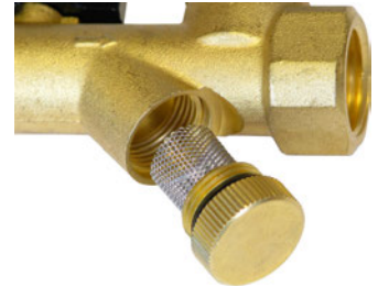
Грязевой фильтр
